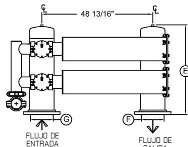
VISTA LATERAL
